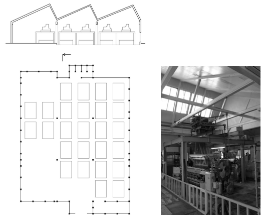
建設時の織機の配置 34) 別工場における稼働中の織機とジャガード 35) 図-4 元来のノコギリ屋根工場内の使い方と別工場で開催している稼働中の織機
